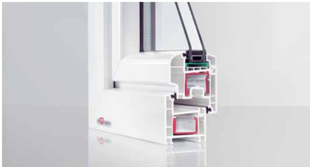
Trīs kameras un 60 mm iebūves dziļums
