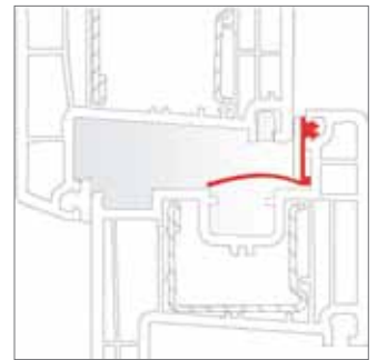
Blīvējuma pozīcija pie normāla gaisa spiediena
