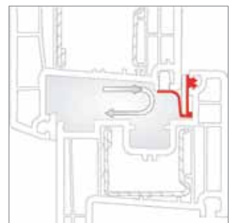
Pieaugot vēja spiedienam, AirComfort sistēma automātiski noslēdzas pēc Bernulli principa
